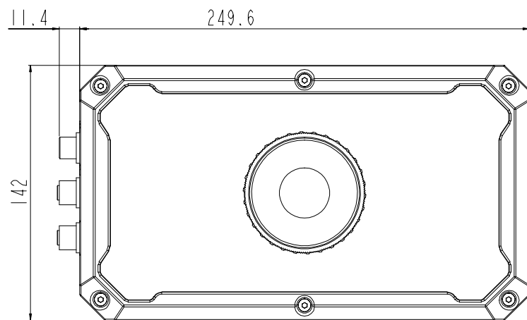
R-8600产品尺寸图
