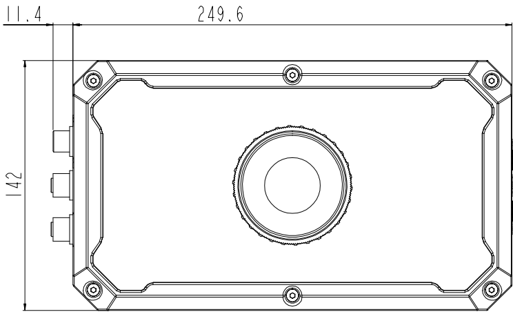
R-8800、R-8120H产品尺寸图
