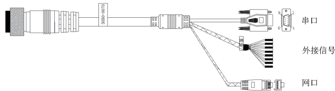
图 1-3 读码器扩展外接功能线定义
