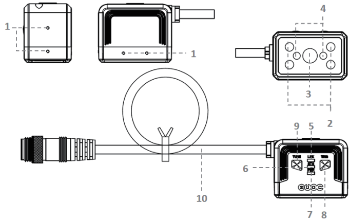
图 1-1 R-R01A07 设备外观
